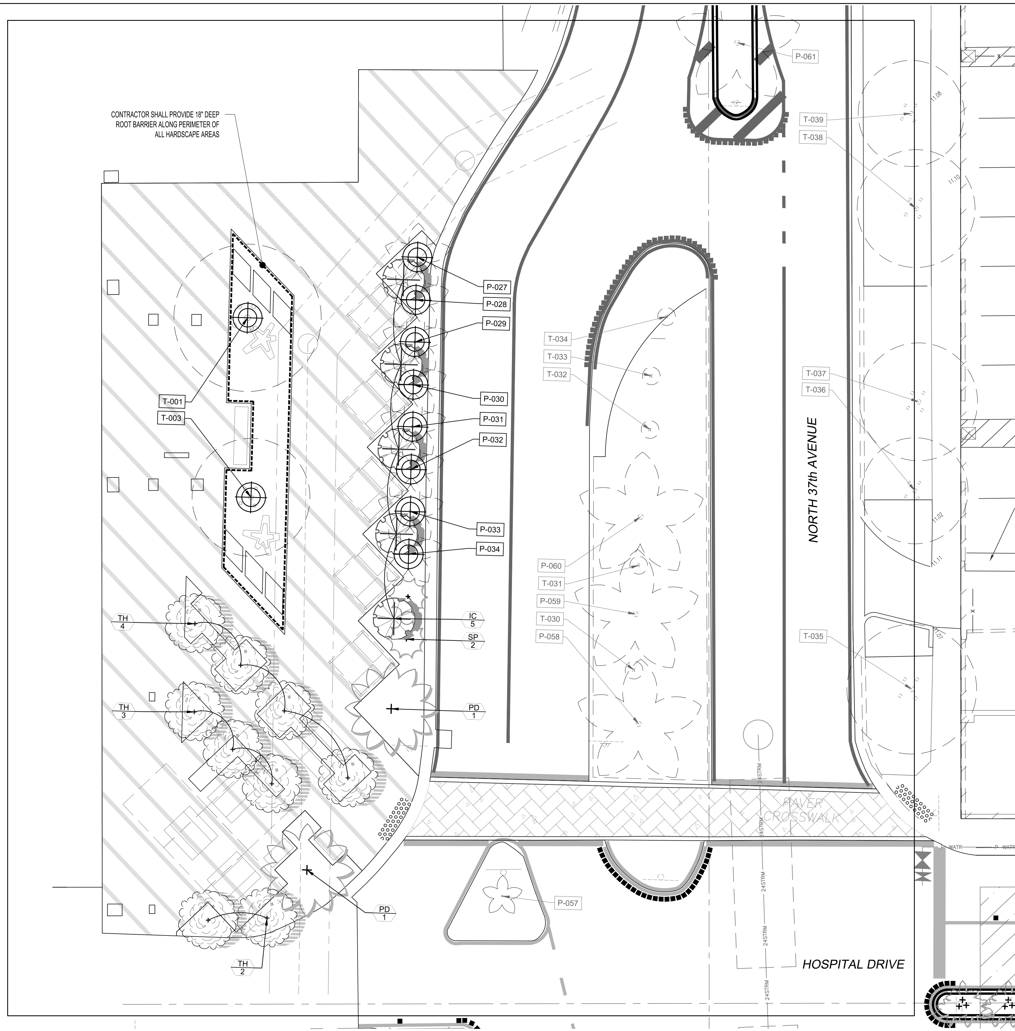
1 ENLARGEMENT PLAN: CORNER PLAZA - CANOPY PLAN
