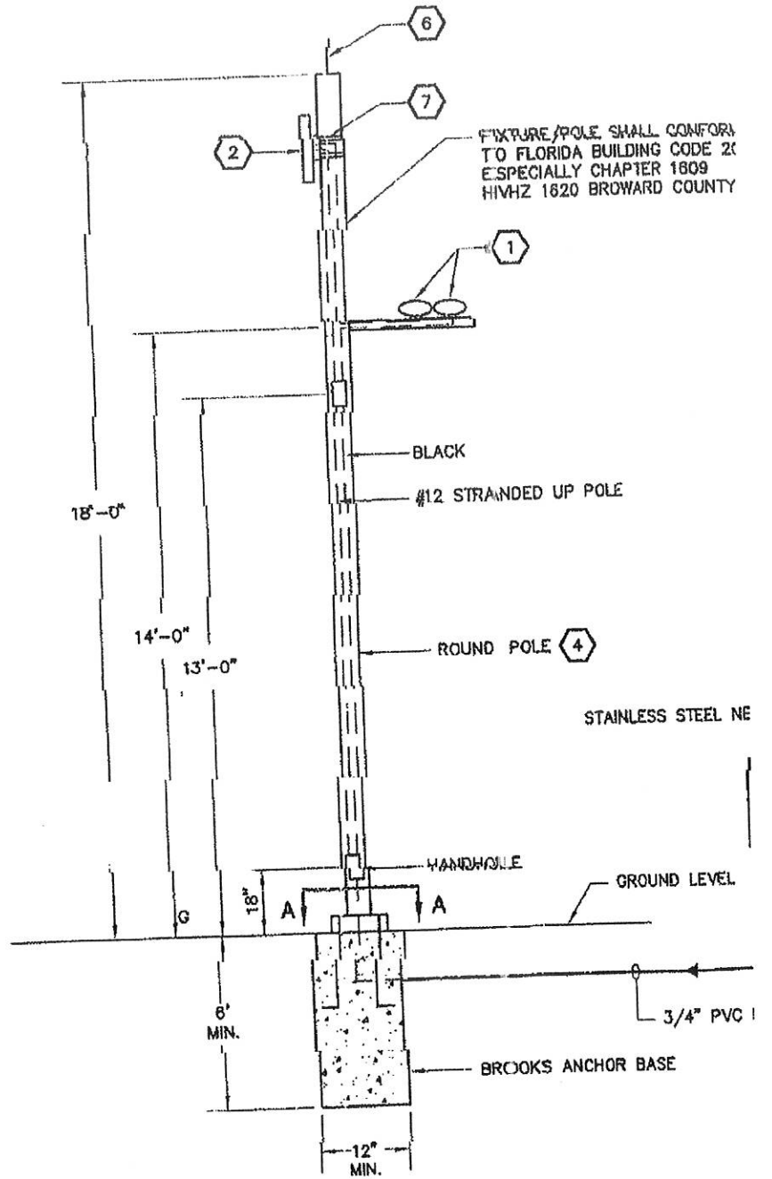
METAL CAMERA POLE DETAIL N.T.S.
