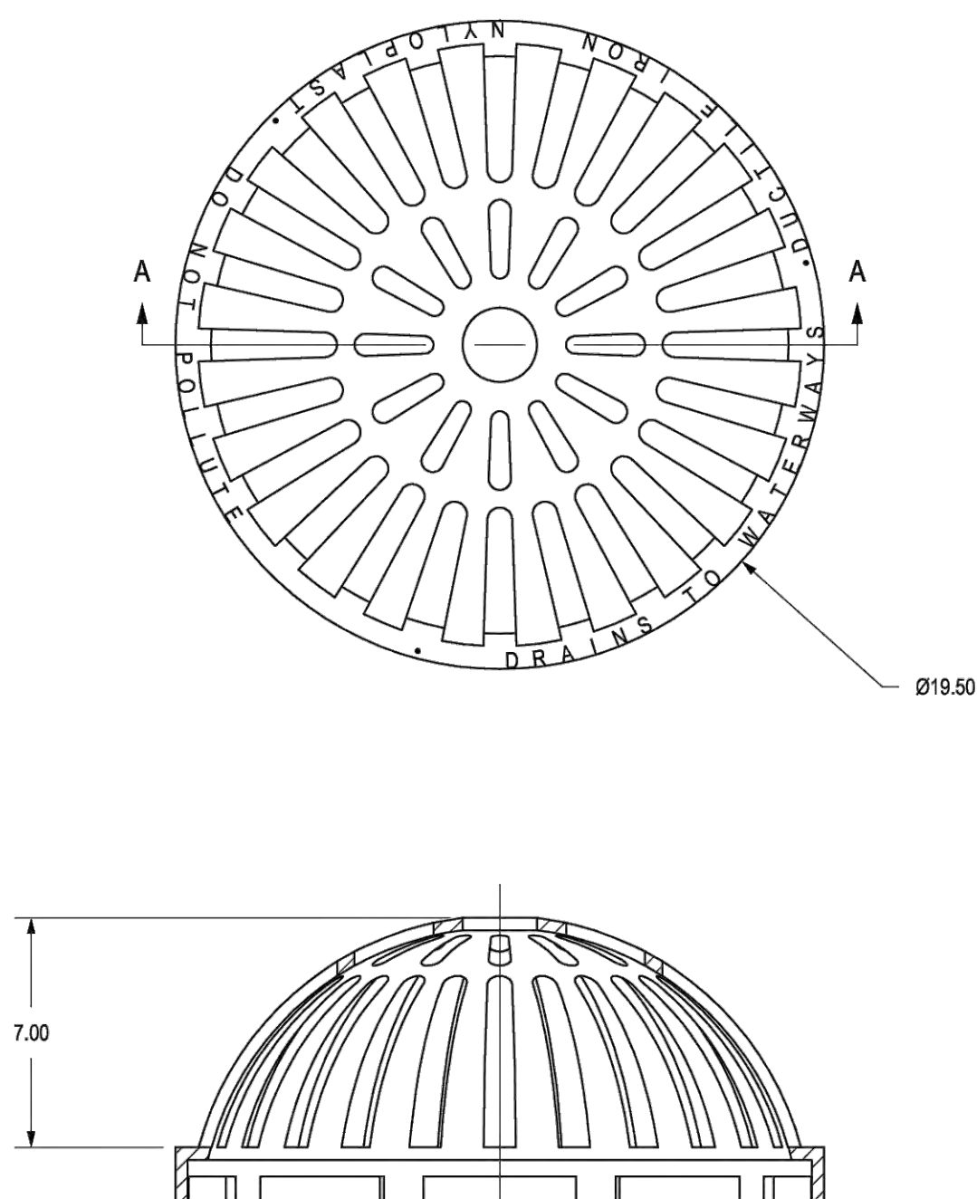
SECTION A-A
